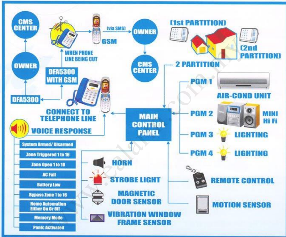
DFA5300 16 ZONES
