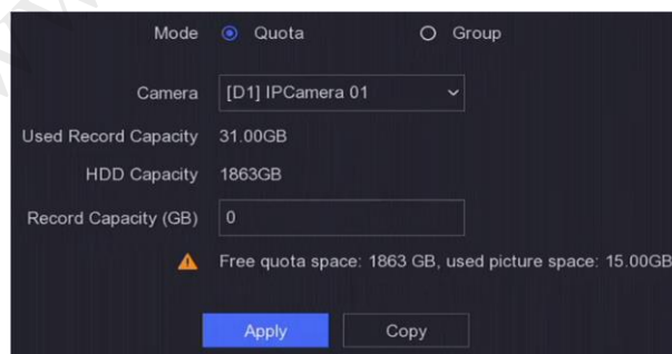
Figure 6-28 Quota
